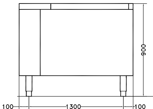
Oldalnézet
