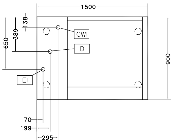
Felülnézet
